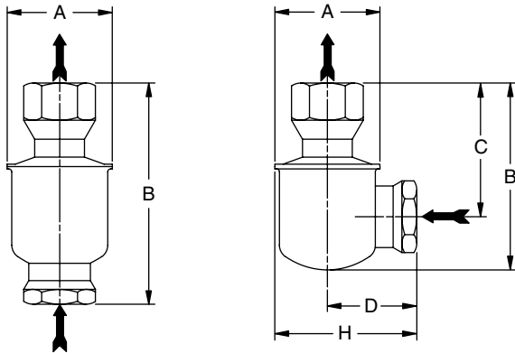
TTF-1 Durchgangsanschluss
